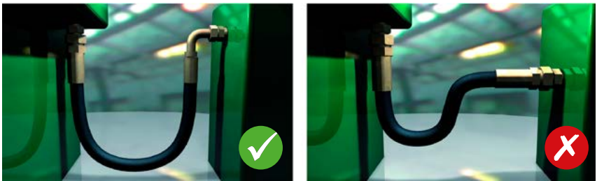
Abb. 8 Biegeradius
