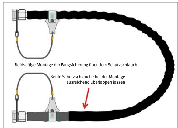
Abb. 19 Überlappende Schutz- schläuche bei beidseitiger Befestigung mit Fangsicherung
