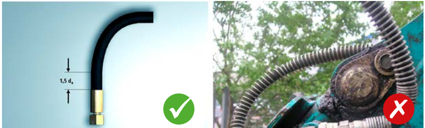
Abb. 9 Richtig: Gerader Abschnitt mit 1,5 d_s vor Biegung Falsch: Eine Schlauchscheuerschutzspirale stellt keinen Knickschutz dar
